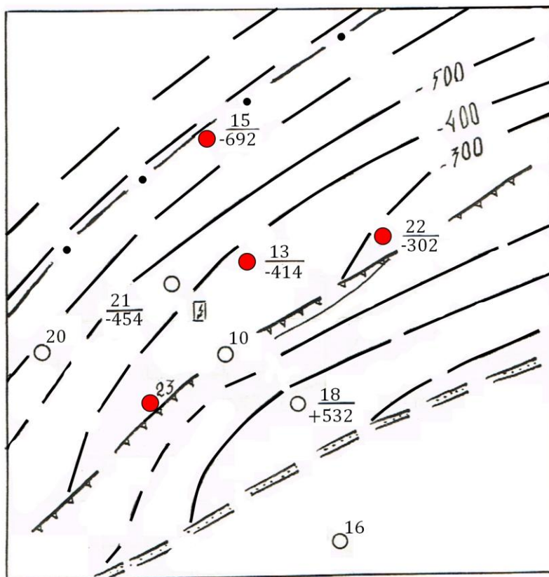
Рисунок 1 – Схематическая структурная карта месторождения Оби-Шифо
