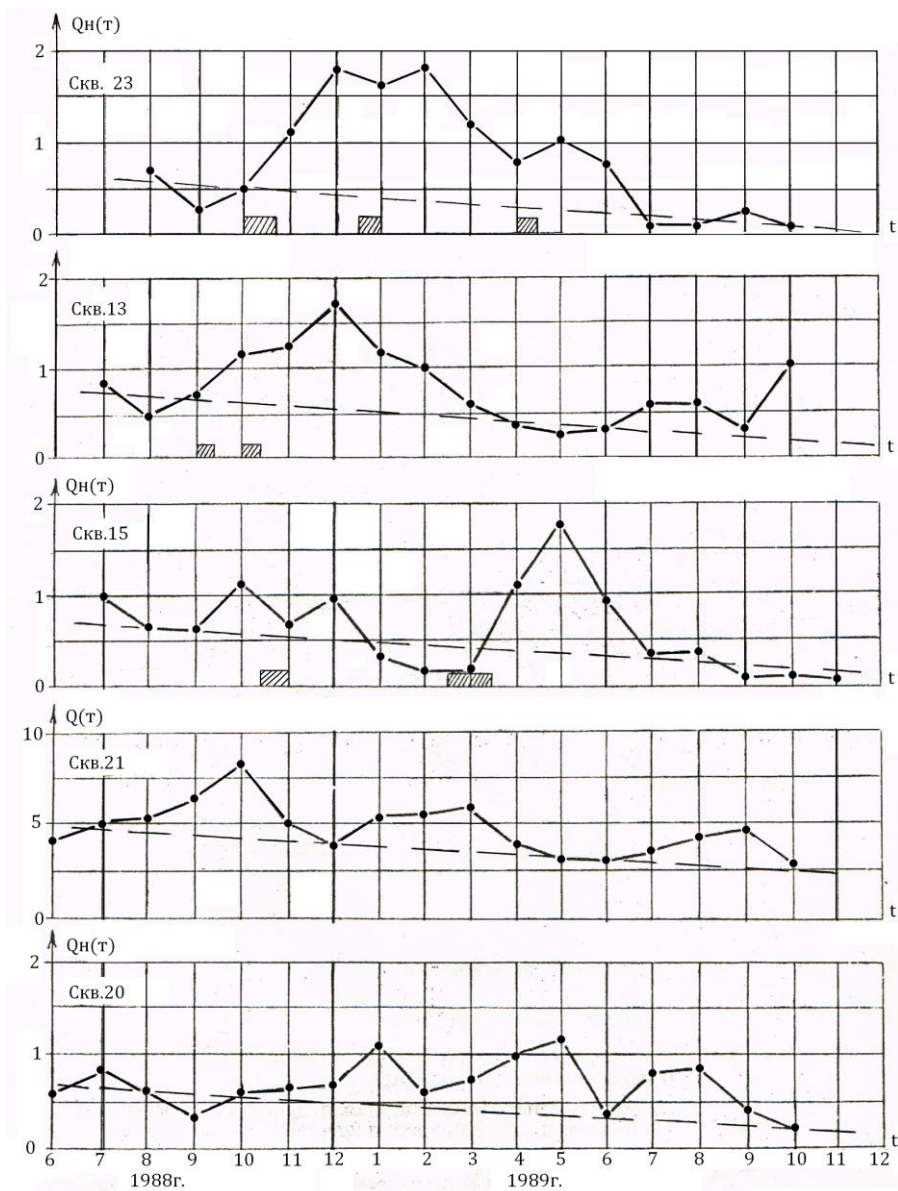
Рисунок 2 – Результаты воздействия электрическим полем на пласт в скважинах месторождения Оби-Шифо (Таджикнефть)
