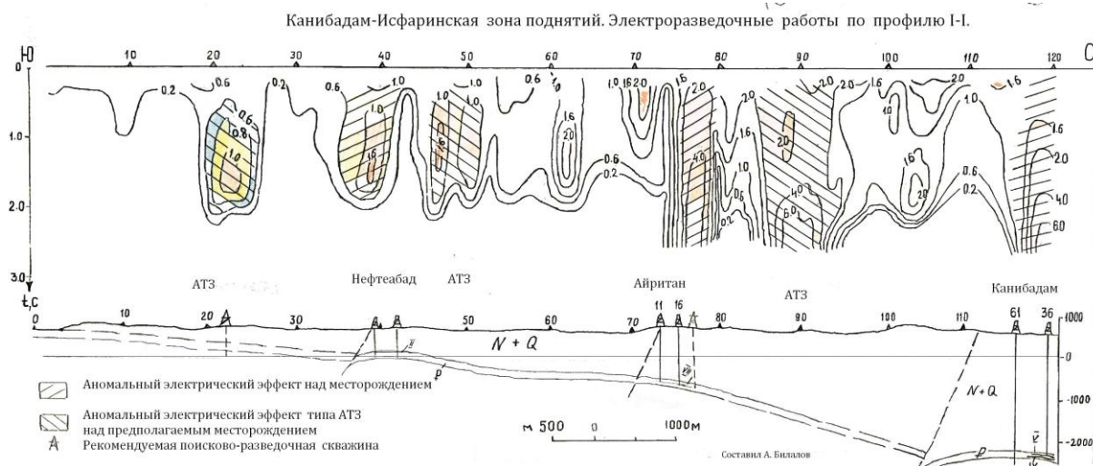
Рисунок 1 – Канибадам-Исфаринский зона поднятий. Электроразведочные работы по профилю I-I
