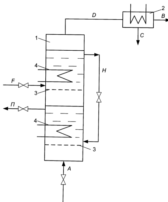
Рисунок 2 – Схема двухзонного реактора: 1 - реактор, 2 – конденсатор, 3 - непроваляные тарелки с колпачковыми, клапанными или ситчатыми газораспределительными устройствами, 4 – нагревающие элементы, А – газообразный агент, В – газообразная фракция, С – углеводородная фракция, D – парогазовая смесь, F – исходные отходы, H – жидкая смесь углеводородов, П – легколетучие углеводороды
