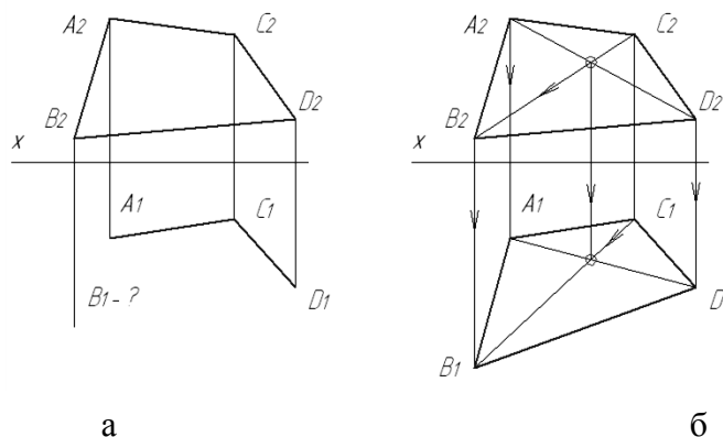
Рисунок 2 - Построение недостающей проекции вершины плоскости: а – условие задачи, б – решение задачи.
