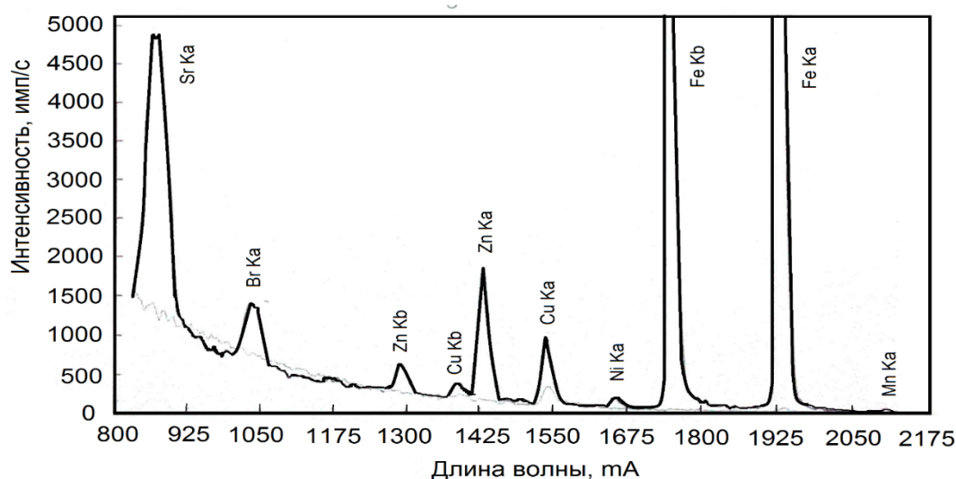
Рисунок 1 – Спектр рентгеновской флуоресценции неорганической части плотного осадка нефтесодержащего шлама УПН «Баган» ООО «ЛУКОЙЛ-Коми»
